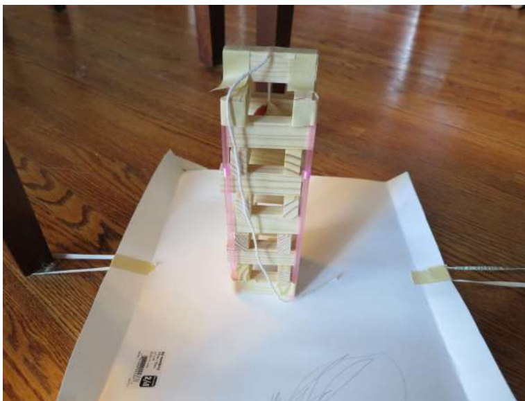
Tour renforcée à l'aide de pailles avec un pendule à l'intérieur.
